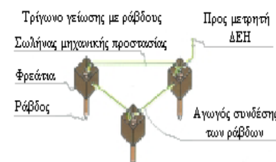
Γειωτής τριγώνου
